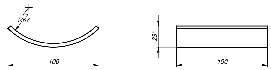
Поз.2 (Ложемент)
